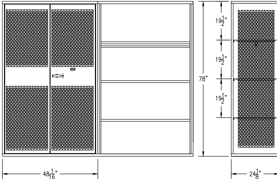
ELEVATION
