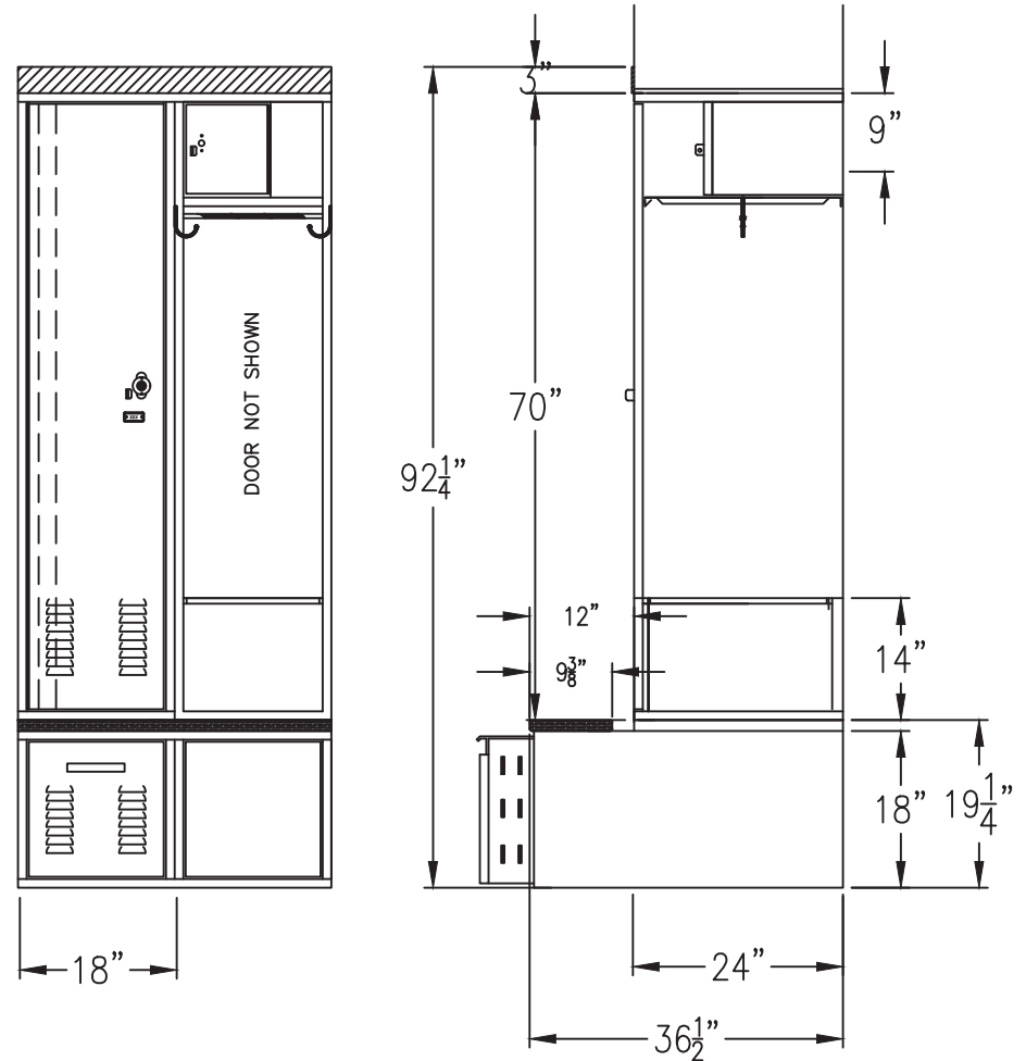
ELEVATION
